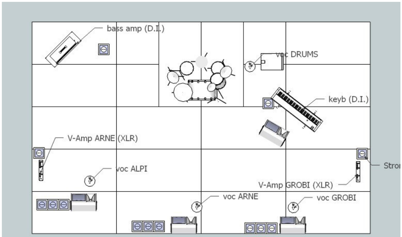
STAGEPLAN (SCHEMATISCH) AUF BEISPIEL-BÜHNE (8 * 5 M)
